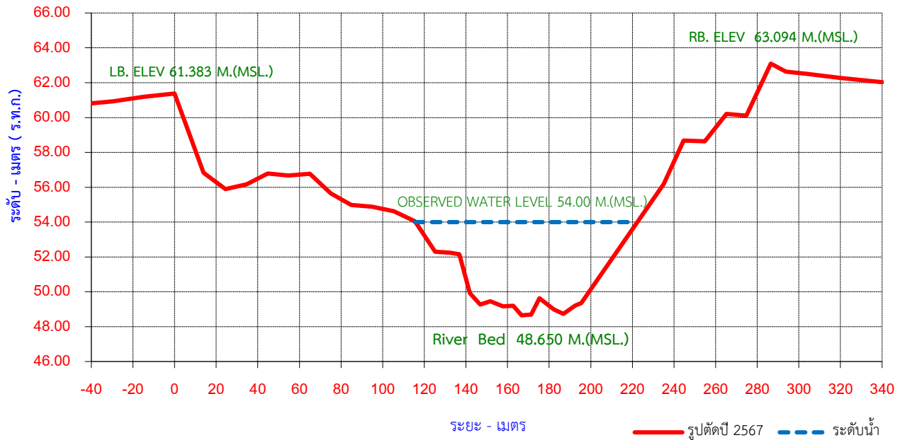
รูปตัดขวางลำน้ำ ปีน้ำ 2567 สถานี N.2B แม่น้ำน่าน อ.เมือง จ.อุตรดิตถ์
